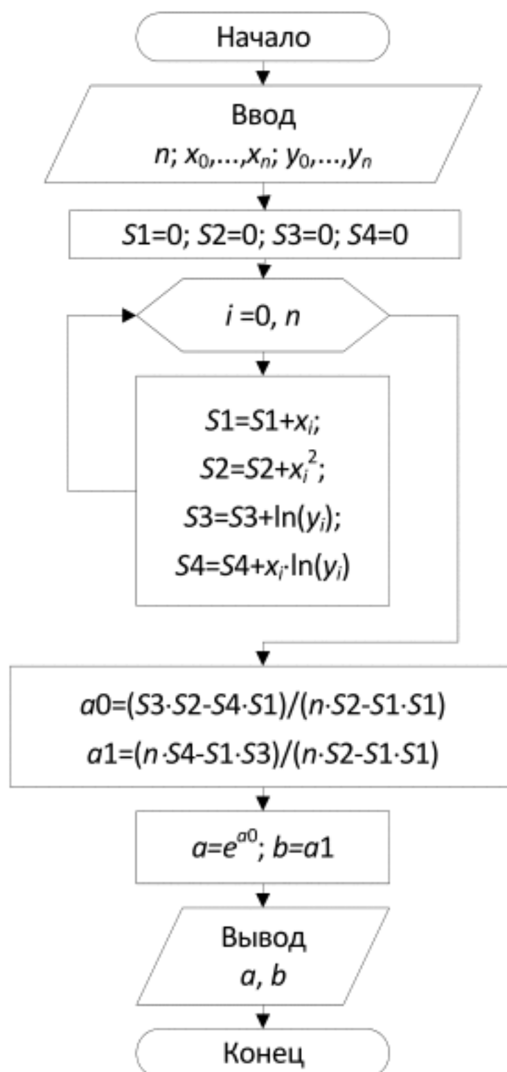
Рис. 5.11. Блок-схема аппроксимации показательной функцией
