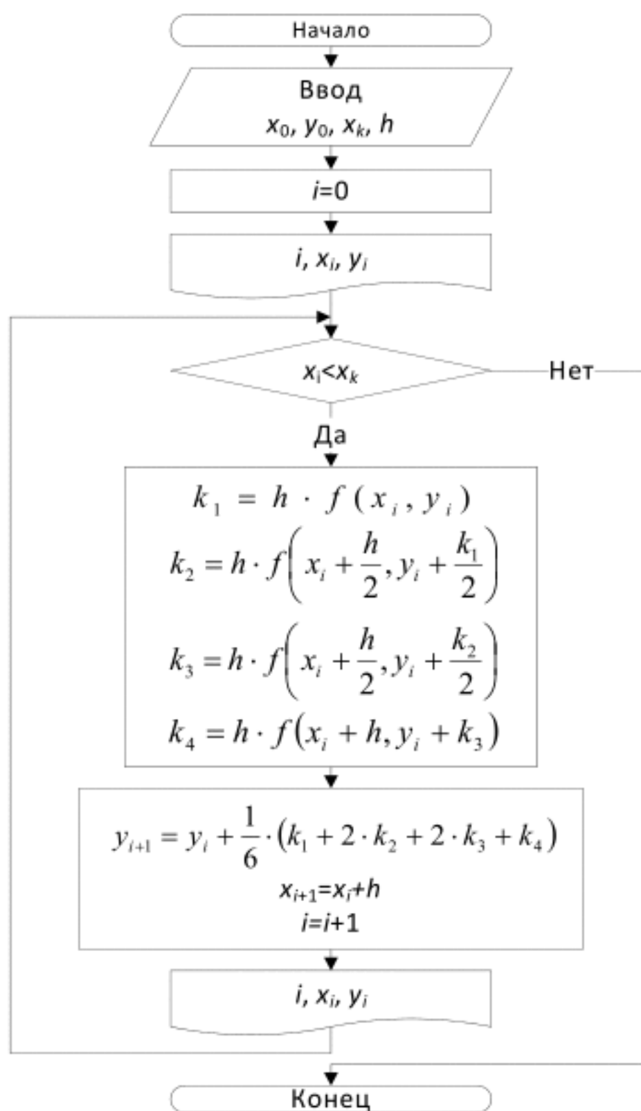
Рис. 8.7. Блок-схема метода Рунге–Кутты
