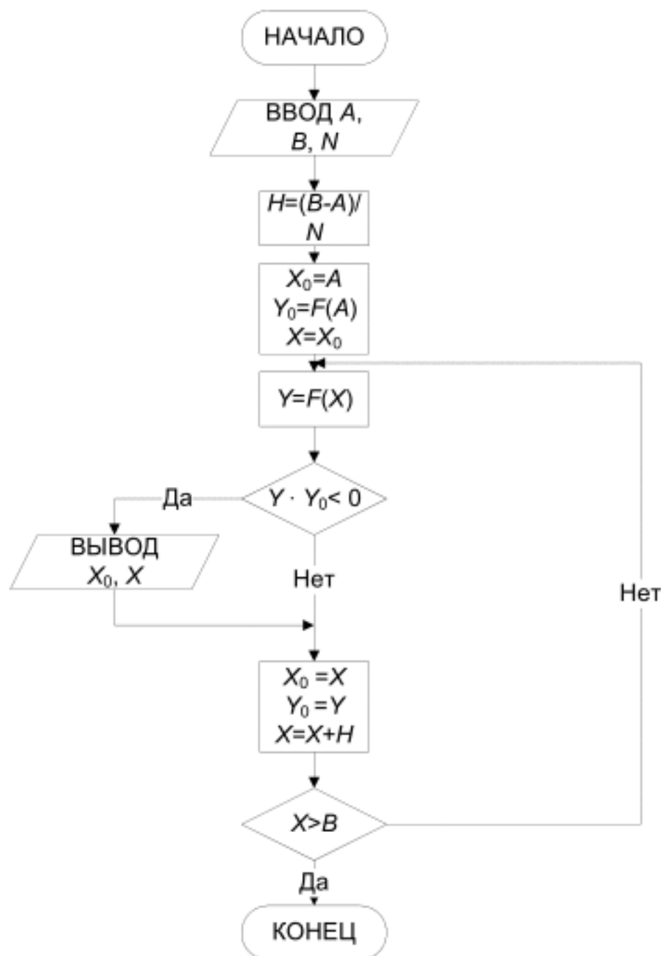
Рис. 2.4. Блок-схема метода отделения корней
