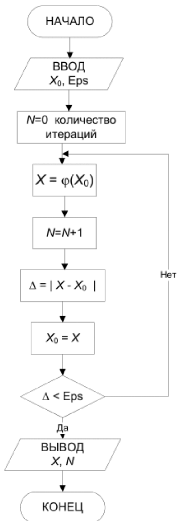
Рис. 2.11. Блок-схема метода простых итераций
