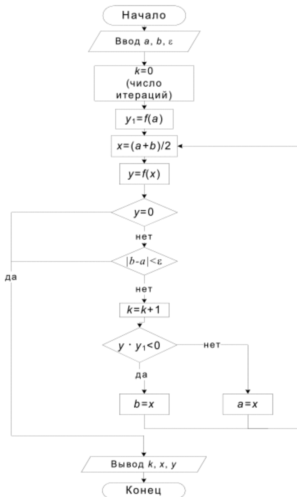
Рис. 2.6. Блок-схема алгоритма метода деления отрезка пополам
