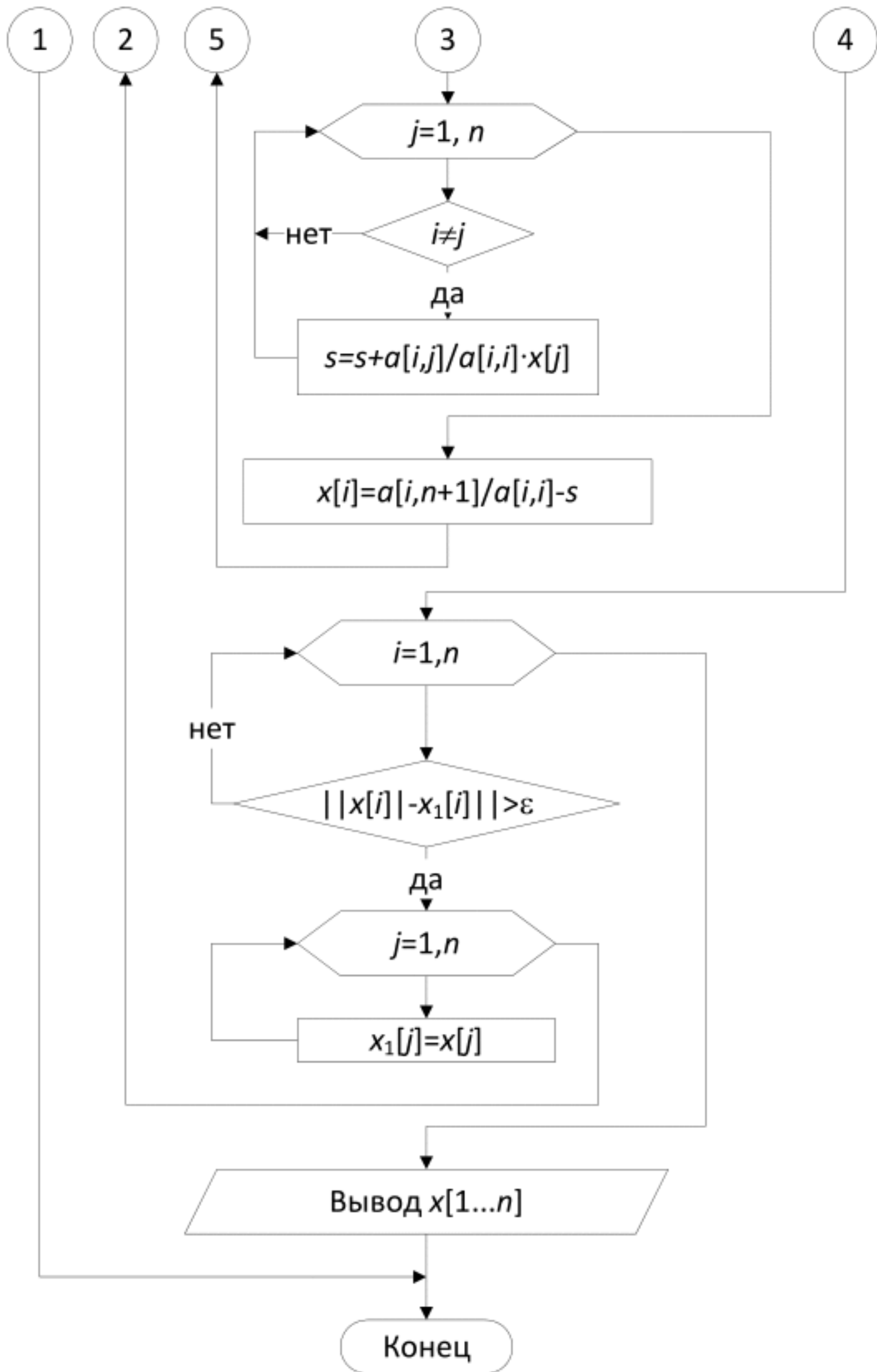
Рис. 3.2. Блок-схема решения системы линейных уравнений методом Гаусса–Зейделя
