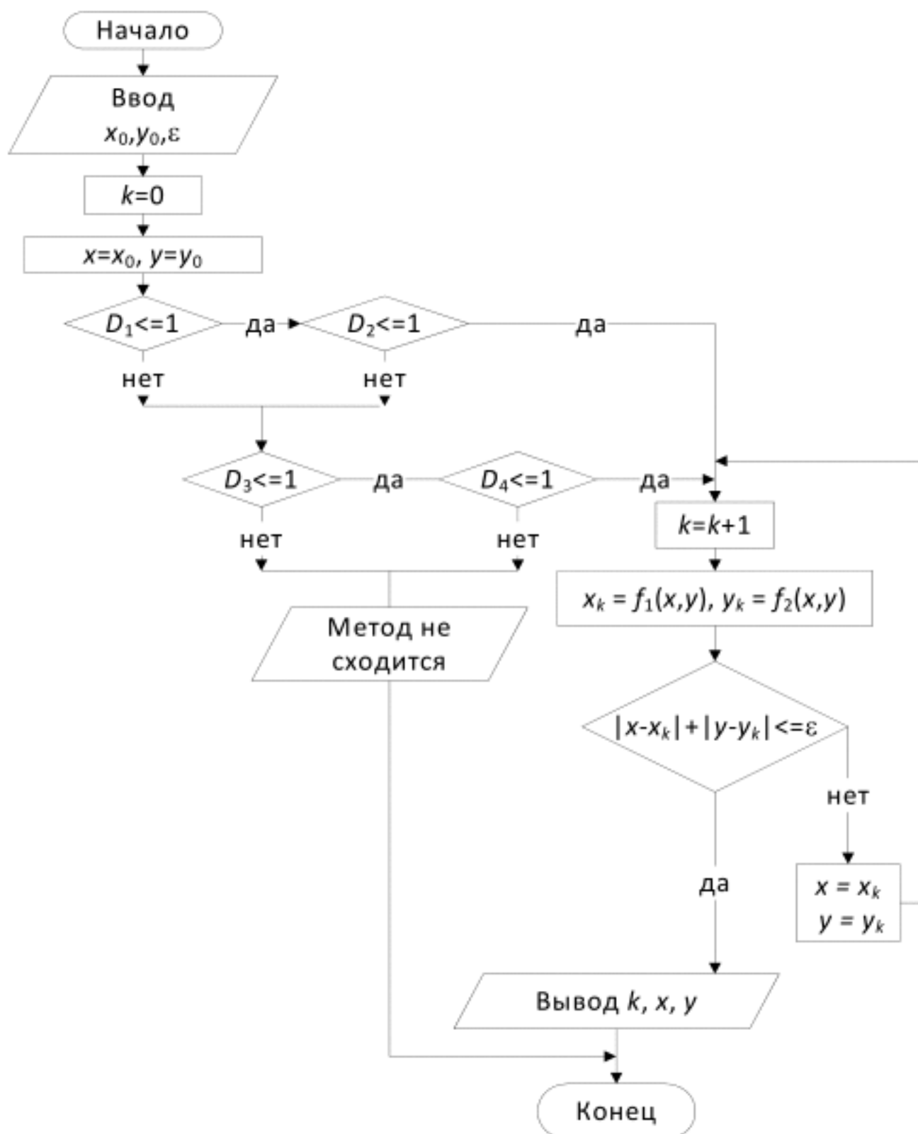
Рис. 4.2. Блок-схема метода простых итераций
