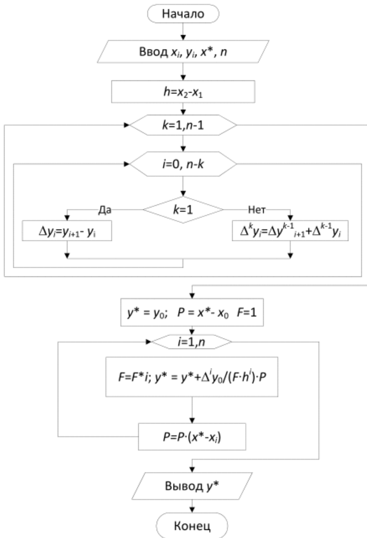
Рис. 5.3. Блок-схема алгоритма метода Ньютона для интерполирования «вперед»
