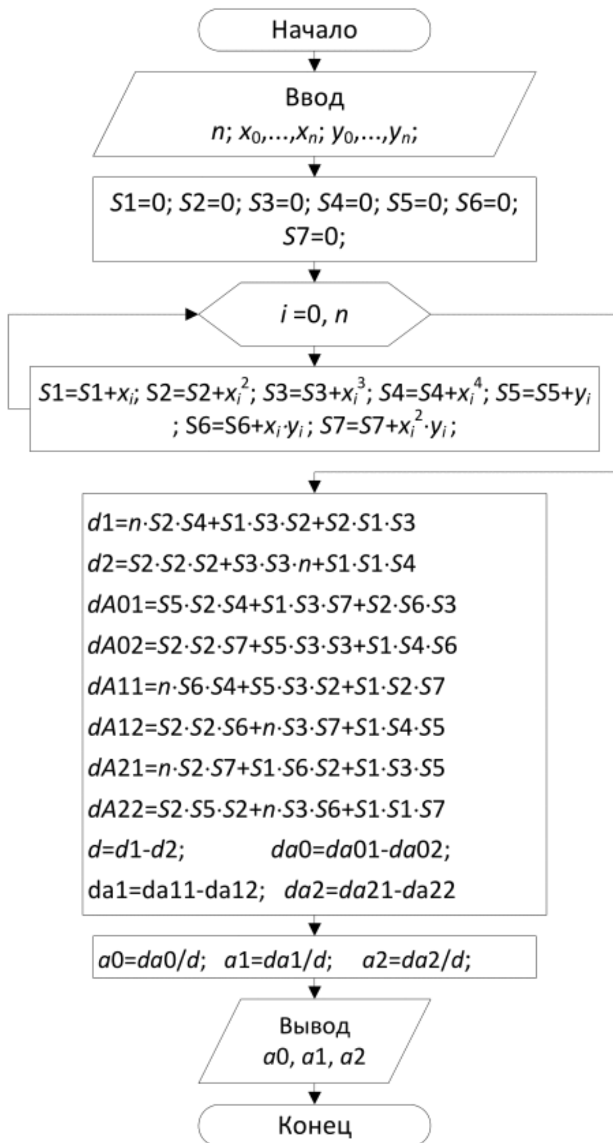
Рис. 5.10. Блок-схема параболической аппроксимации
