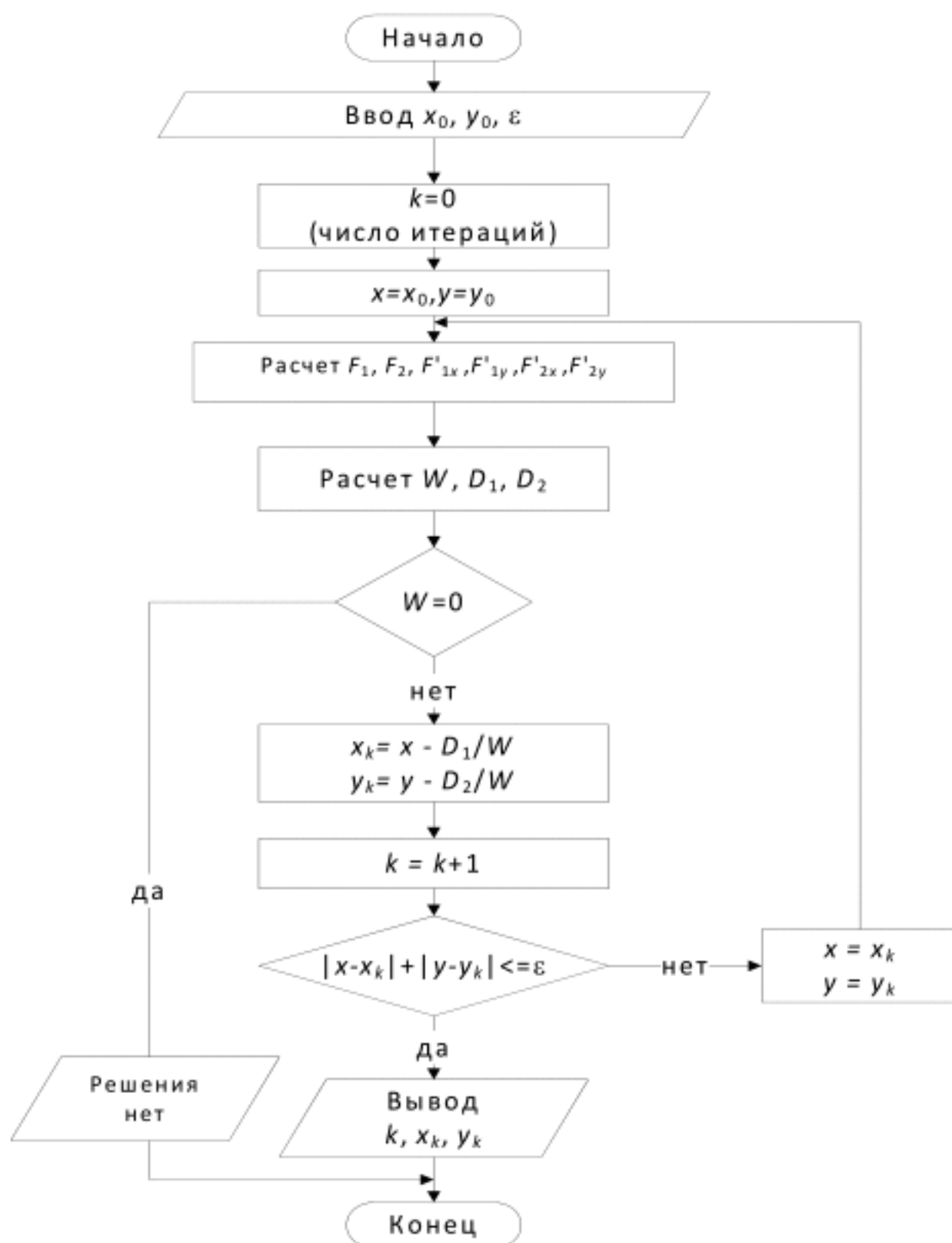
Рис. 4.3. Блок-схема метода Ньютона
