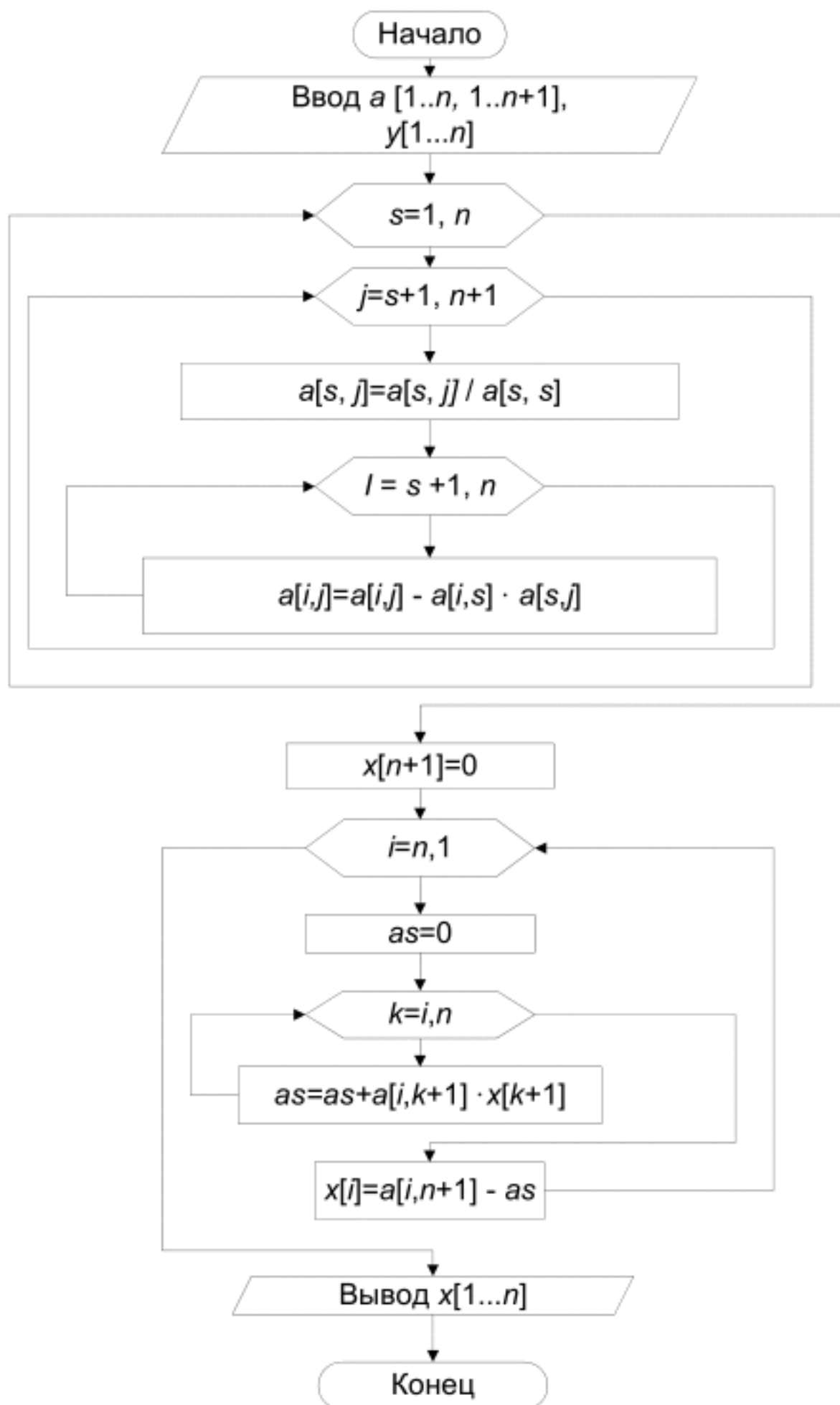
Рис. 3.1. Блок-схема метода Гаусса
