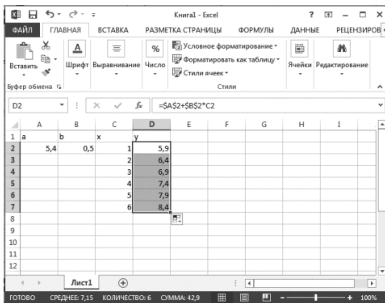
Рис. 9.5. Копирование формулы
