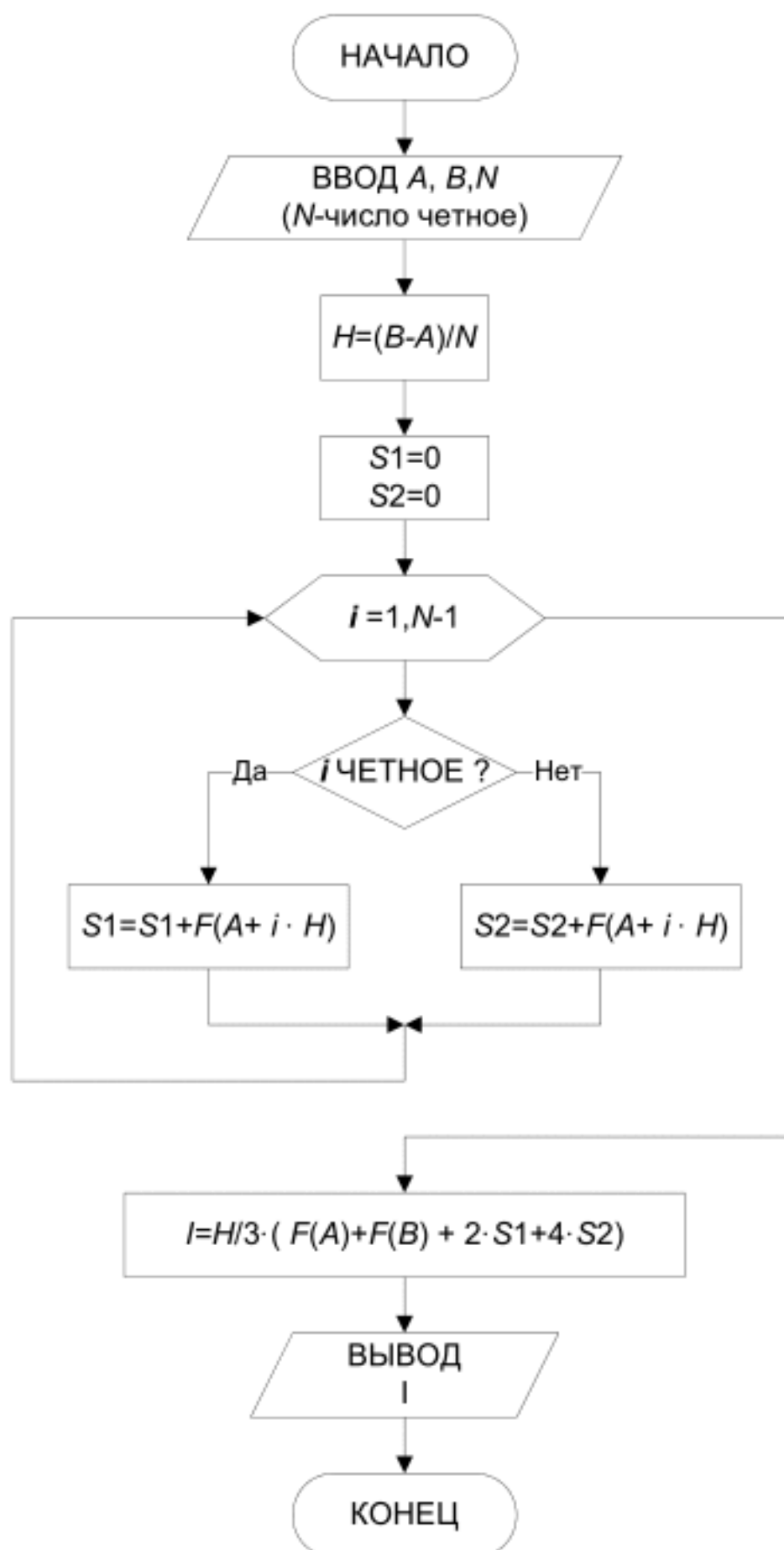
Рис. 7.8. Блок-схема метода Симпсона
