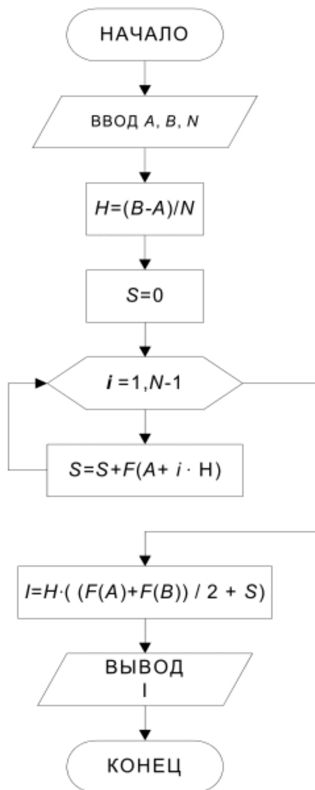
Рис. 7.6. Блок-схема метода трапеций
