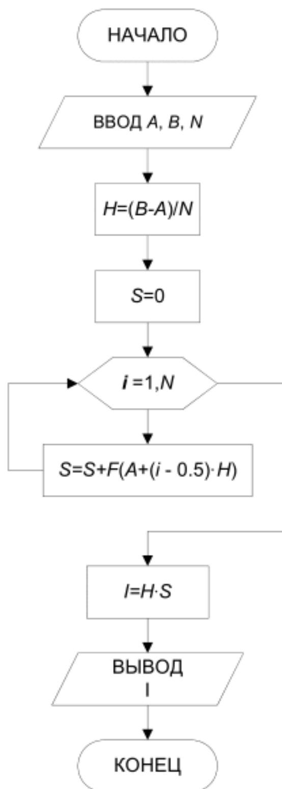
Рис. 7.3. Блок-схема метода прямоугольников
