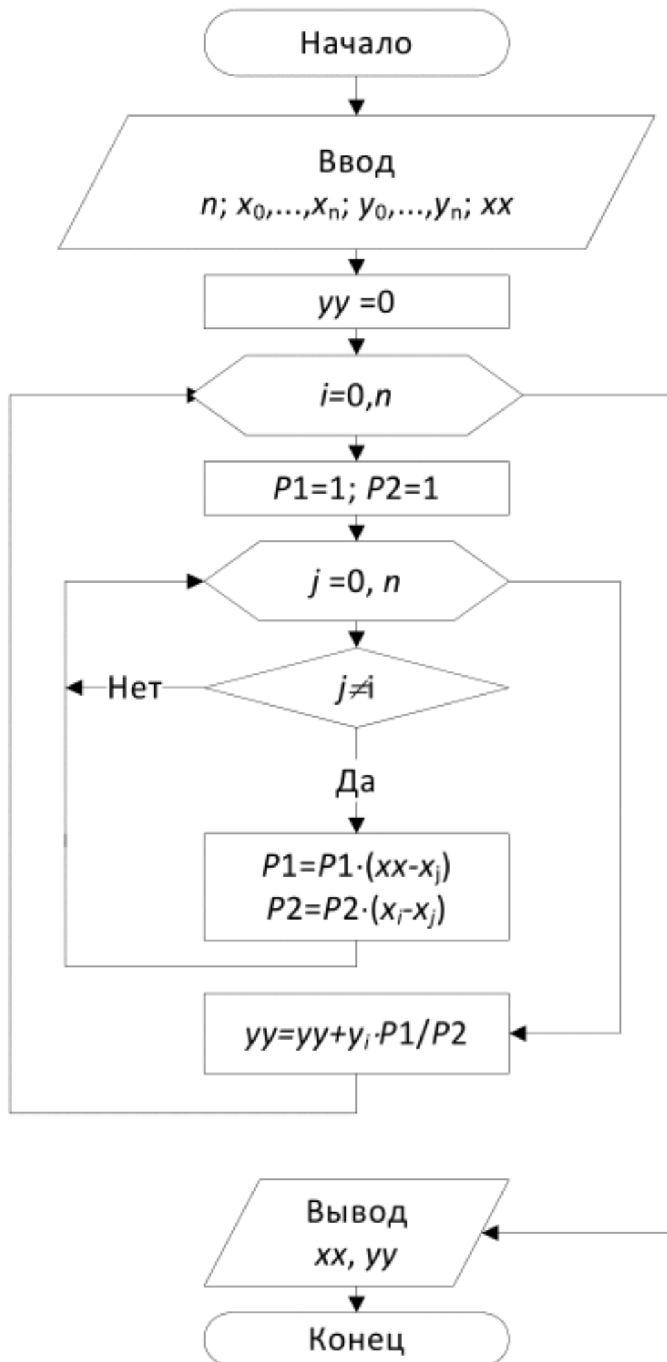
Рис. 5.2. Блок-схема метода Лагранжа
