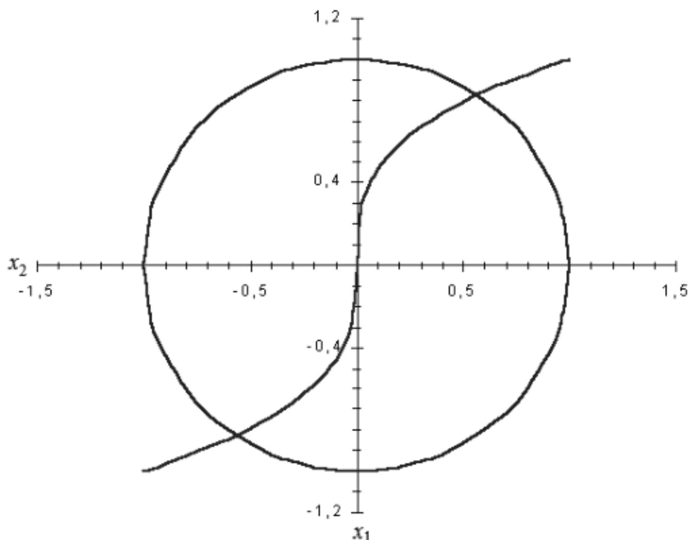
Рис. 4.1. Отделение корней системы нелинейных уравнений
