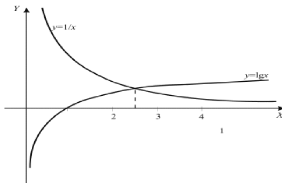
Рис. 2.1. Графический метод отделения корней
