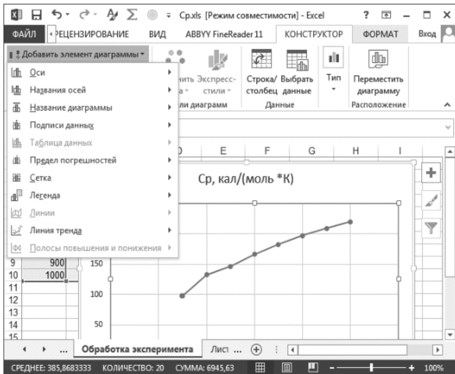
Рис. 9.15. Оформление диаграммы
