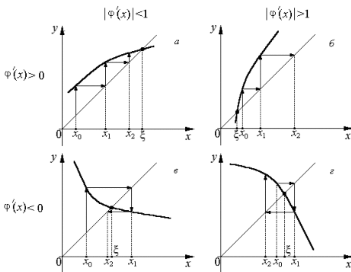
Рис. 2.10. Метод простых итераций
