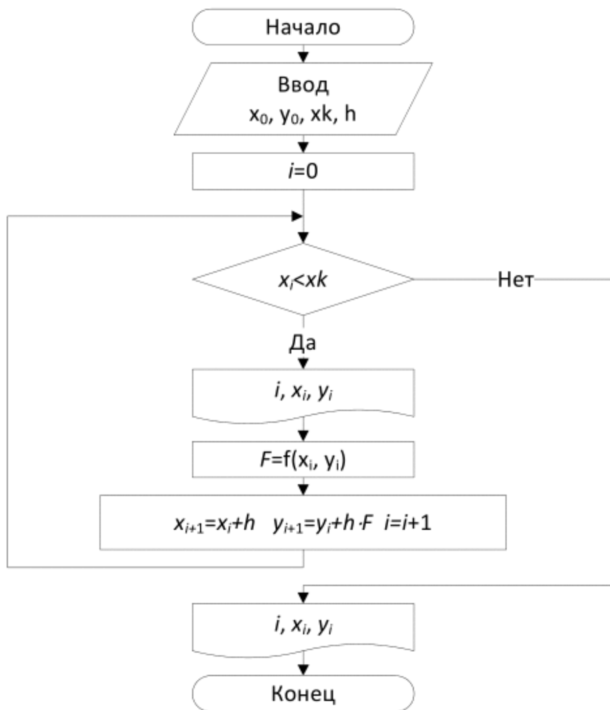
Рис. 8.2. Блок-схема метода Эйлера
