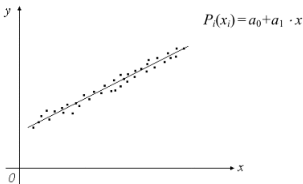
Рис. 5.7. Линейная аппроксимация
