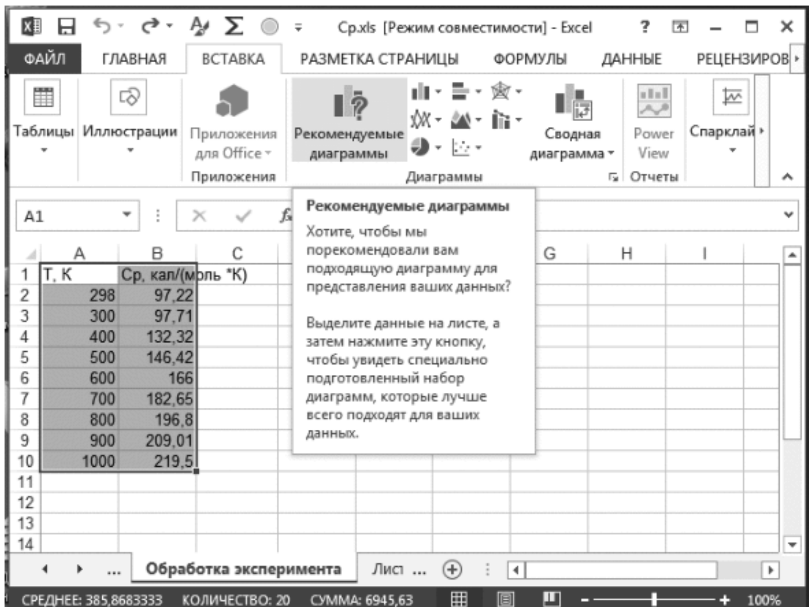
Рис. 9.13. Построение диаграмм
