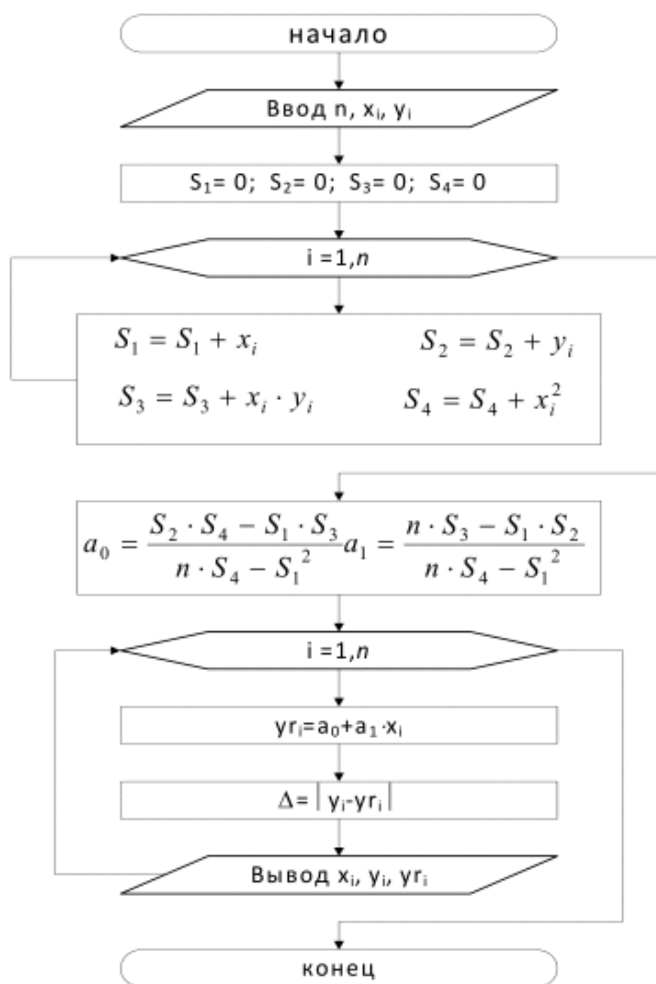
Рис. 5.8. Блок-схема линейной аппроксимации
